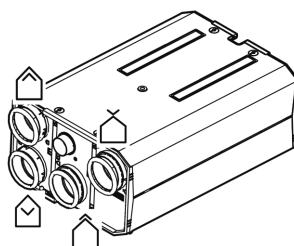
podlahová montáž
